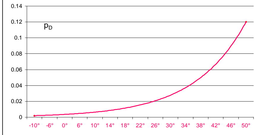
饱和压力是气体温度的函数
