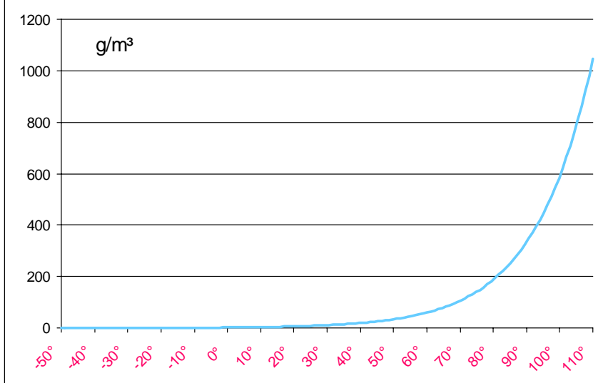
空气的含水能力也是温度的函数
